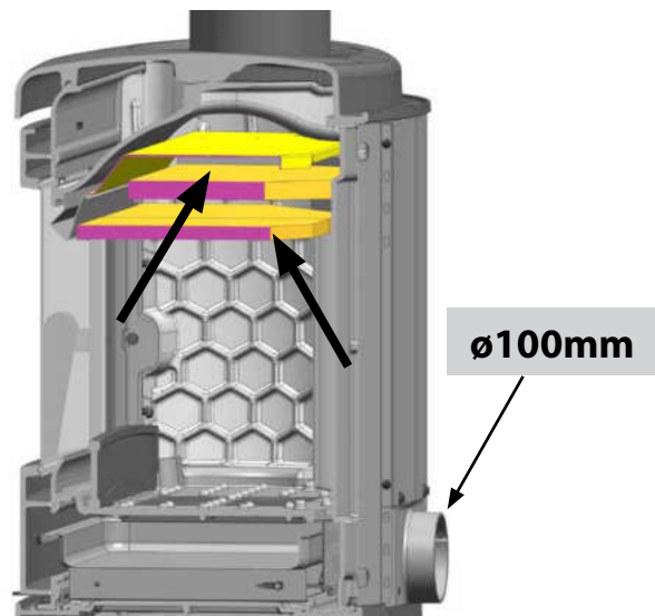
DEFLETTORE FUMO SMOKE DEFLECTOR RAUCHUMLENKPLATTE DÉFLECTEUR FUMÉE DEFLECTOR DE HUMO
